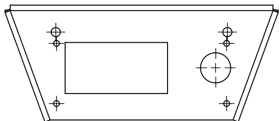
1 x Cache écran LCD
